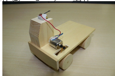
工作② モーター工作
